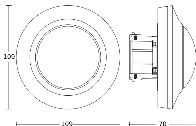
Dessin dimensionnel 1
